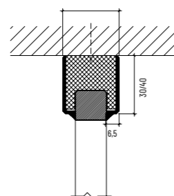
Spoj so stropom
