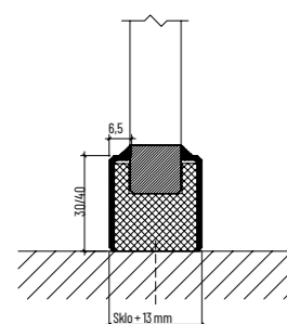
Spoj s podlahou
