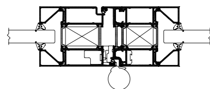
Sklenené dvere s hliníkovým rámom
