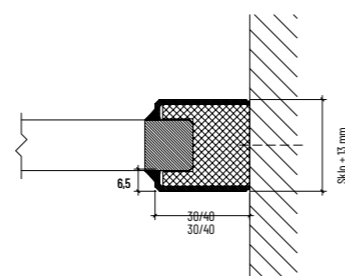
Spoj so stenou
